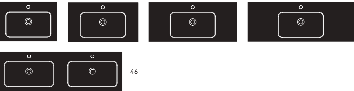
Bowl's depth / Profondeur de la vasque: 12 cm / Basin's thickness / Épaisseur de la vasque: 2.5 cm Bowl's width / Largeur de la vasque: 50cm (for basin/pour vasque 60-80-100-120) / 45cm (for basin/pour vasque 120 twin/double)
