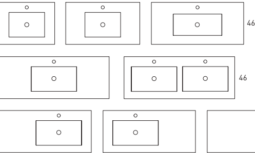
Bowl's depth / Profondeur de la vasque: 17 cm / Basin's thickness / Épaisseur de la vasque: 1.8 cm / Bowl's width / Largeur de la vasque: 46 cm
